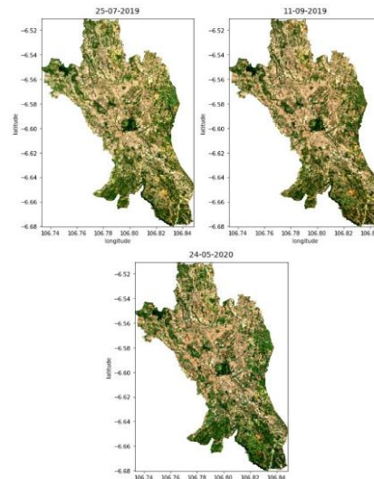
Gambar 4. Kota Bogor Tanpa Awan
