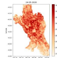
Gambar 7. Peta Sebaran Suhu Udara
