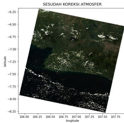
Gambar 2. Koreksi Atmosfer Citra Landsat
