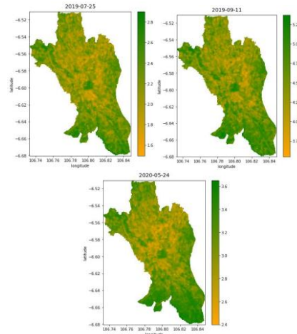
Gambar 11. Peta Sebaran Evapotranspirasi Aktual
