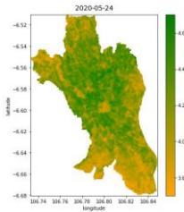
Gambar 9. Peta Sebaran Evapotranspirasi Potensial
