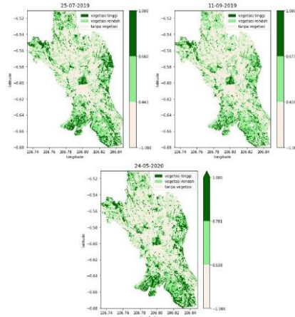
Gambar 5. Peta Sebaran Vegetasi
