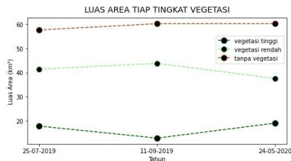
Gambar 6. Perbandingan Luas Area Vegetasi
