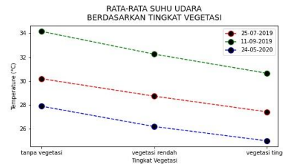
Gambar 8. Perbandingan Suhu Udara
