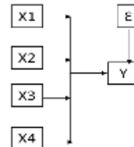
Gambar 5b. Model Hubungan Linier Berganda
