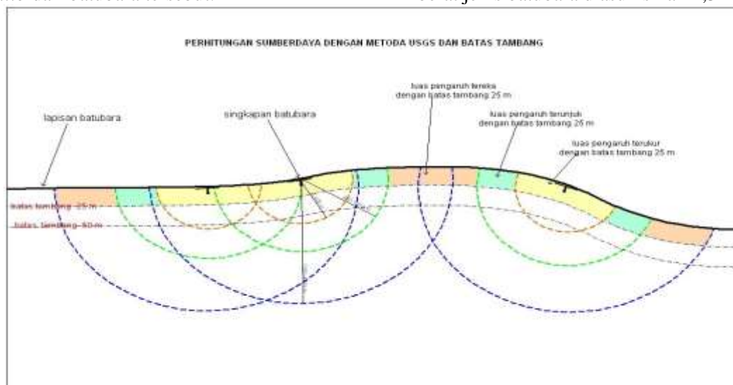
Gambar 4. Perhitungan sumber daya berdasarkan metoda USGS- Circular 891 kategori terukur, terunjuk, dan tereka yang dibatasi oleh kedalaman tambang.
