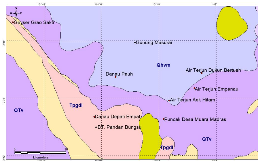
Gambar 1. Satuan Batuan penyusun daerah penelitian, diwakili oleh simbol dan warna (Sumber: Peta Geologi Regional Lembar Sungaipenuh dan Ketaun)
