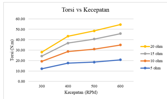
Gambar 4.12 Grafik hasil nilai Torsi (V) dengan variasi beban R dan Kecepatan
