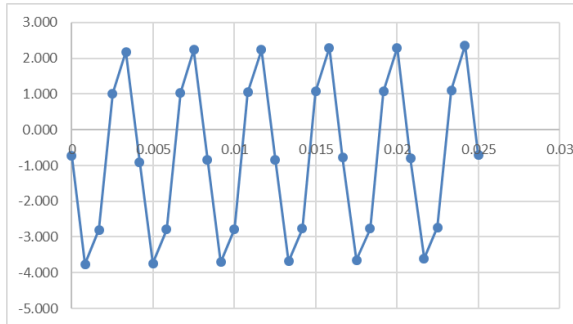
Gambar 6: Grafik Torsi dari Hasil Simulasi 500RPM
