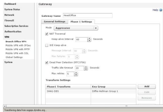
Fig. 16. Gateway VPN
