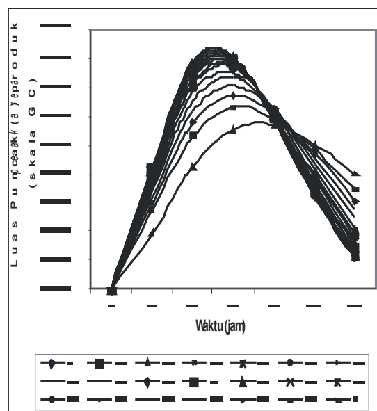
Gambar 8. Grafik hasil simulasi konsentrasi produk melalui pengembangan variabel pH untuk RPM 150
