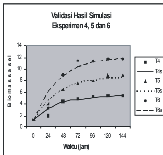
Gambar 5. Kurva validasi hasil simulasi konsentrasi biomassa sel pada Eksperimen 4, 5 dan 6.
