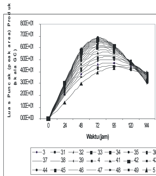
Gambar 7. Grafik hasil simulasi konsentrasi produk melalui pengembangan variabel pH untuk RPM 100
