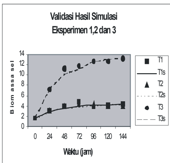
Gambar 4. Kurva validasi hasil simulasi konsentrasi biomassa sel pada Eksperimen 1, 2 dan 3
