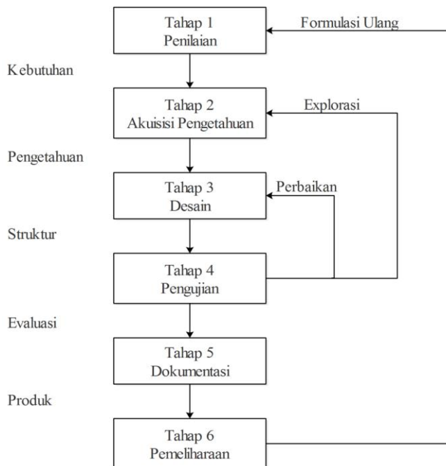
Gambar 1. Tahapan Pengembangan Sistem Pakar [4].
