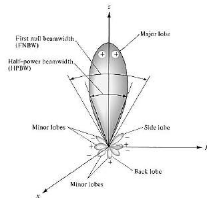
Gambar 2.3. Representasi Pola Radiasi
