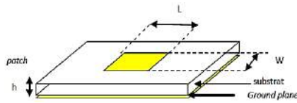
Gambar 2.11. Pola Dasar Antena Planar
