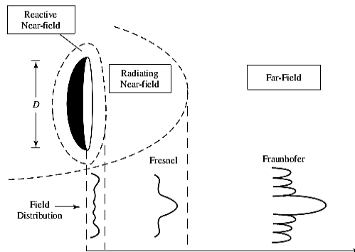
Gambar 2.2. Daerah Radiasi Antena
