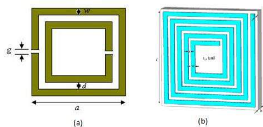
Gambar 2.10. Struktur MNG (a) Struktur Split Ring Resonator (SRR); (b) Struktur Spiral Resonator (SR)
