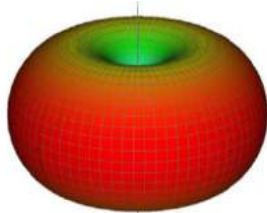
Gambar 2.6. Pola Radiasi Omnidireksional
