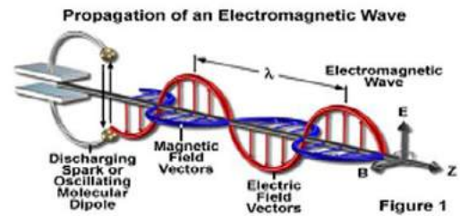
Gambar 2.9. Gelombang Elektromagnetik
