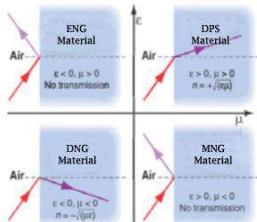
Gambar 2.8. Klasifikasi Material
