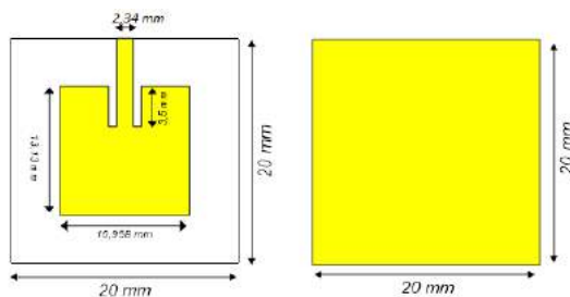
Gambar 3.4. Antena Konvensional; (a) tampak depan, (b) tampak belakang.
